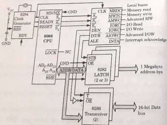
Fig. 3.10.1. Minimum mode 8086 system.
