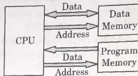
Fig. 1.5.1. Harvard architecture.
