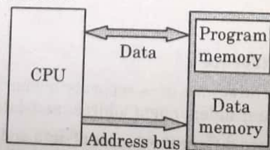
Fig. 1.6.1. Princeton architecture.
