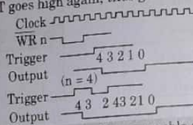
Fig. 5.14.2. Mode 1 : Programmable one-shot.
