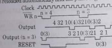
Fig. 5.14.3. Mode 2 : Generator clock.
