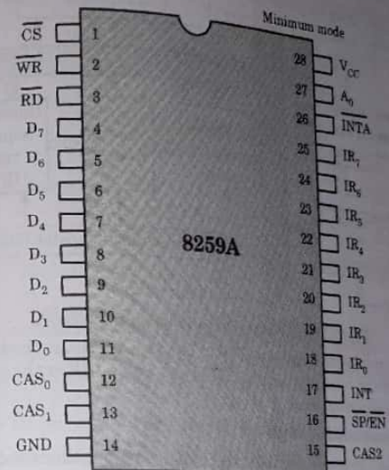
Fig. 5.16.1. 8259A pin diagram.
