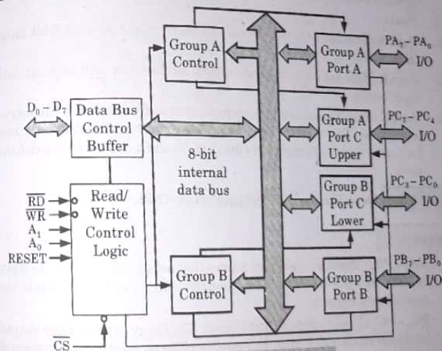
Fig. 5.5.1. 8255 block diagram.
